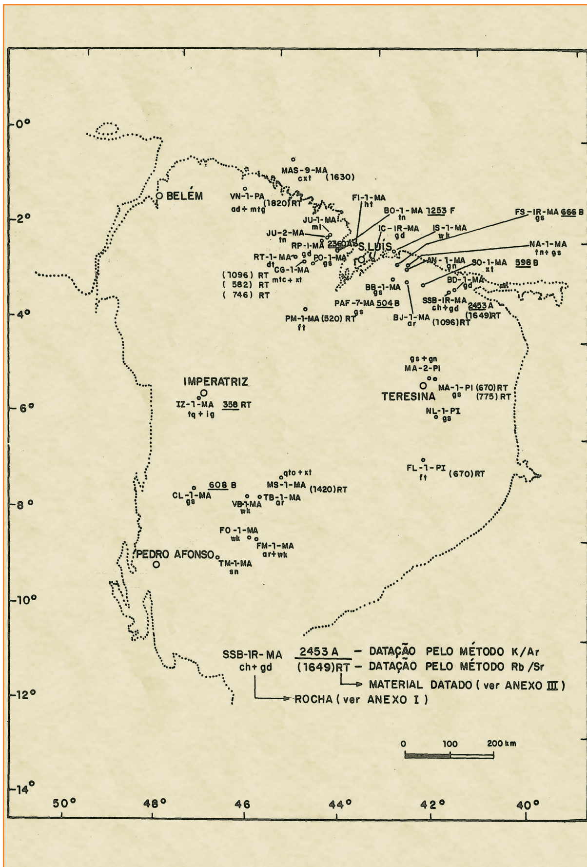
Figura 7 Localização dos poços que atingiram o embasamento, com informações petrográficas e/ou geocronológicas, das Bacias do Maranhão, São Luís e Barreirinhas.
