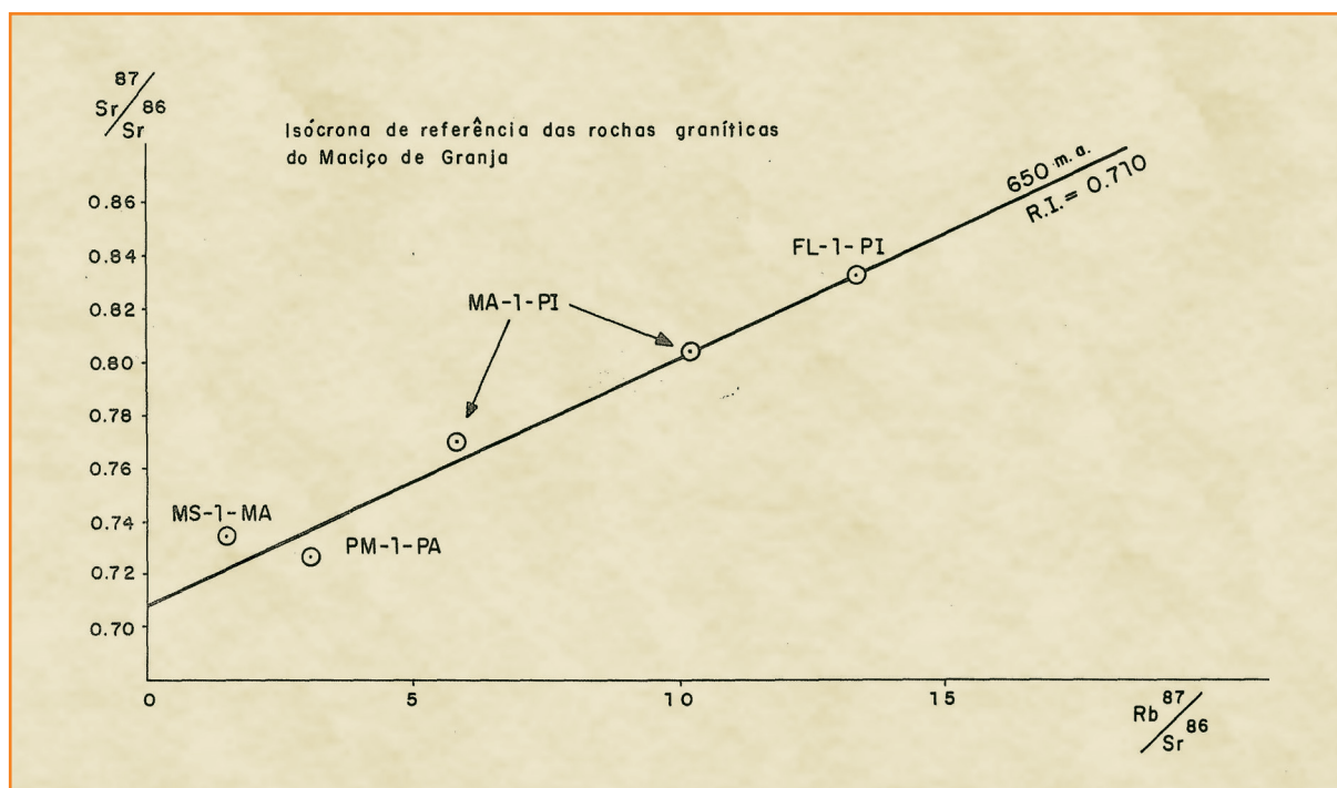
Figura 8 Diagrama isocrônico - rochas do embasamento da Bacia do Maranhão.
