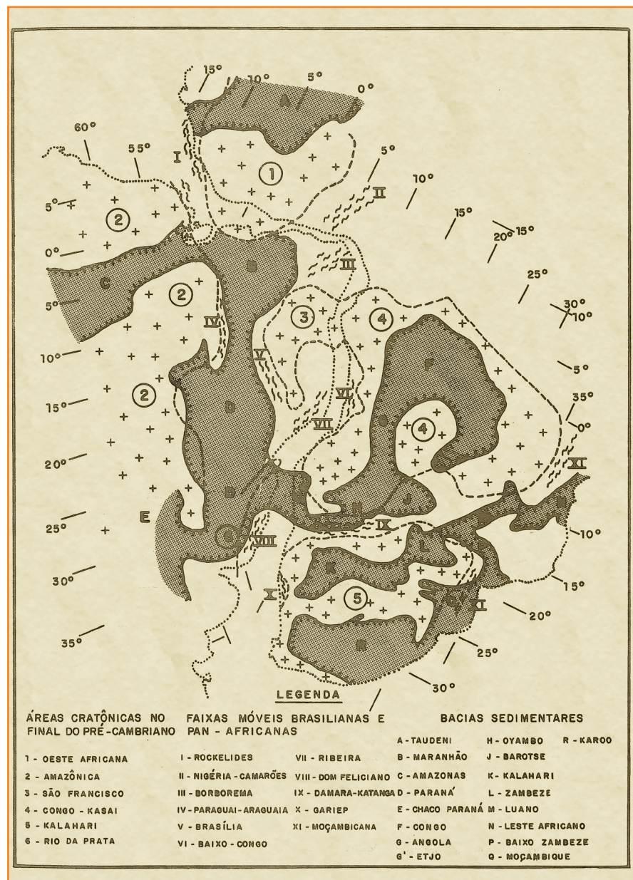
Figura 1 Distribuição geográfica das sinéclises paleozóicas no Gondwana Ocidental.
