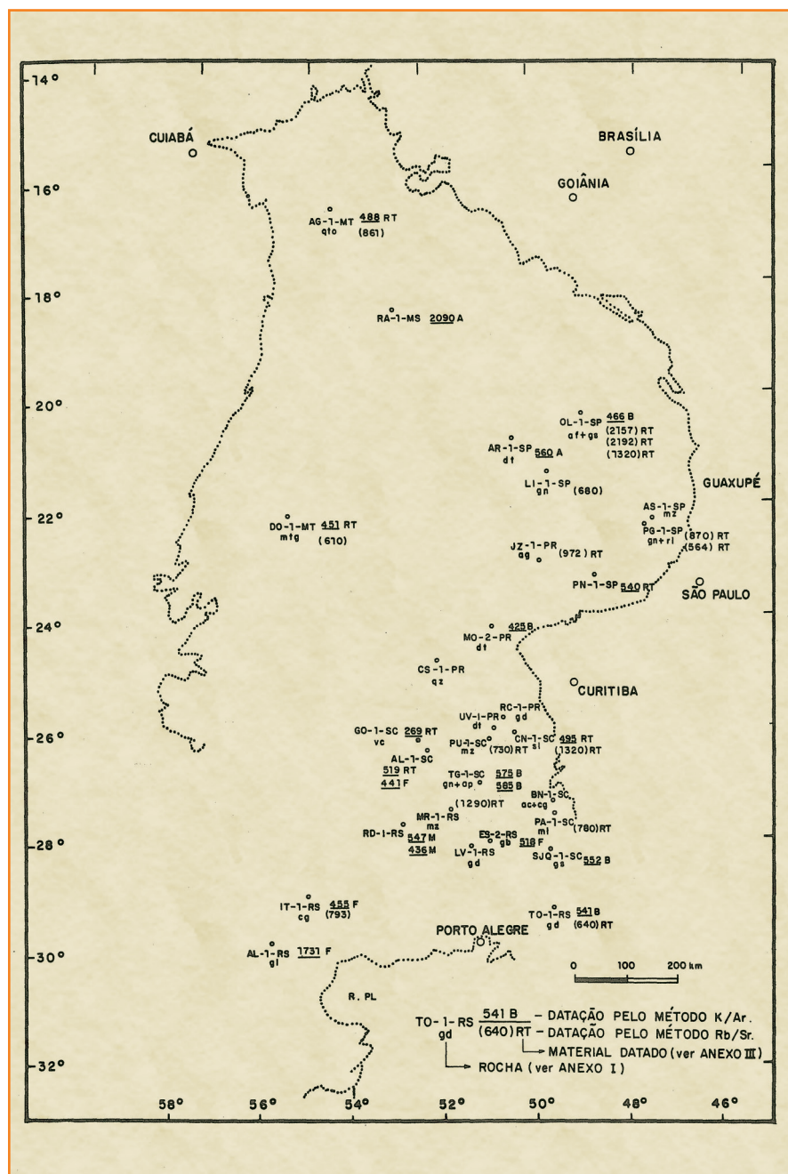
Figura 4 Localização dos poços que atingiram o embasamento, com informações petrográficas e/ou geocronológicas, da Bacia do Paraná.
