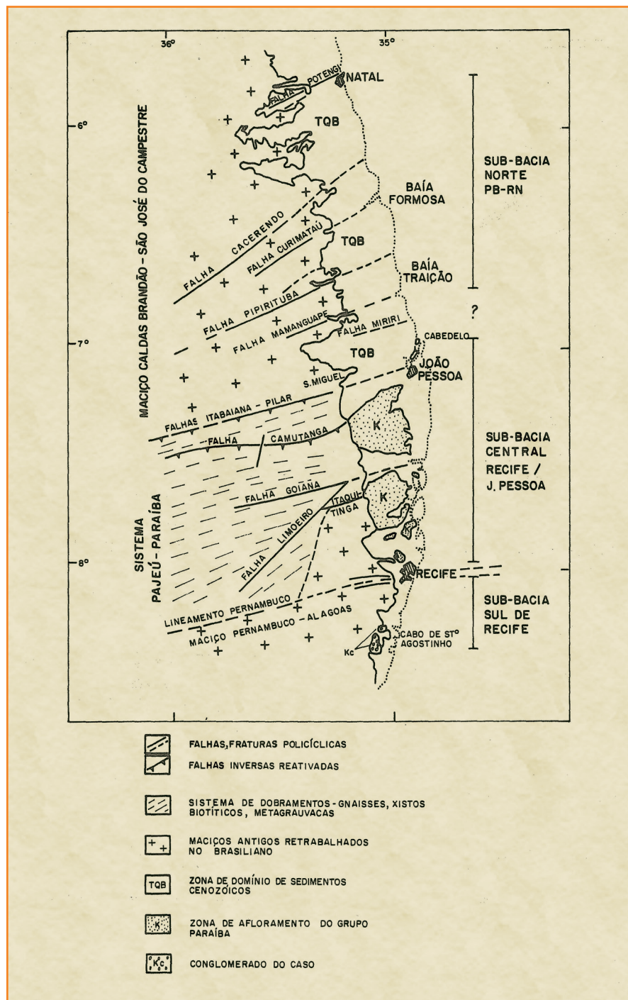
Figura 16 Esquema da estruturação das "Bacias" sedimentares do Saliente Oriental Nordestino.
