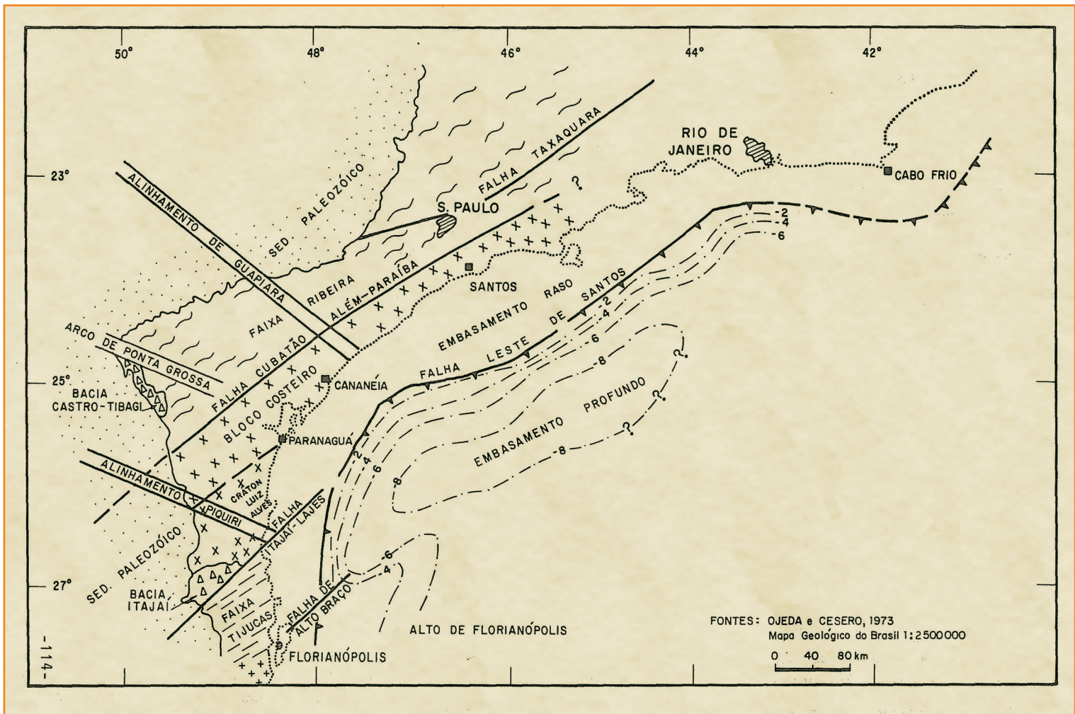
Figura 21 Mapa geológico-geotectônico esquemático do embasamento das Bacias de Santos e Pelotas.
