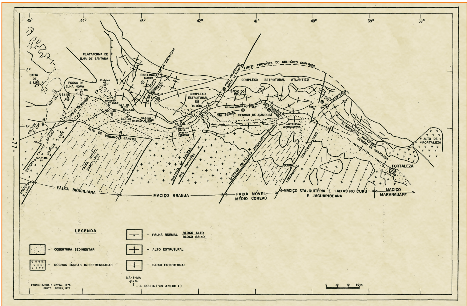
Figura 14 Mapa geológico-geotectônico do embasamento das Bacias de Barreirinhas-Piauí-Ceará.
