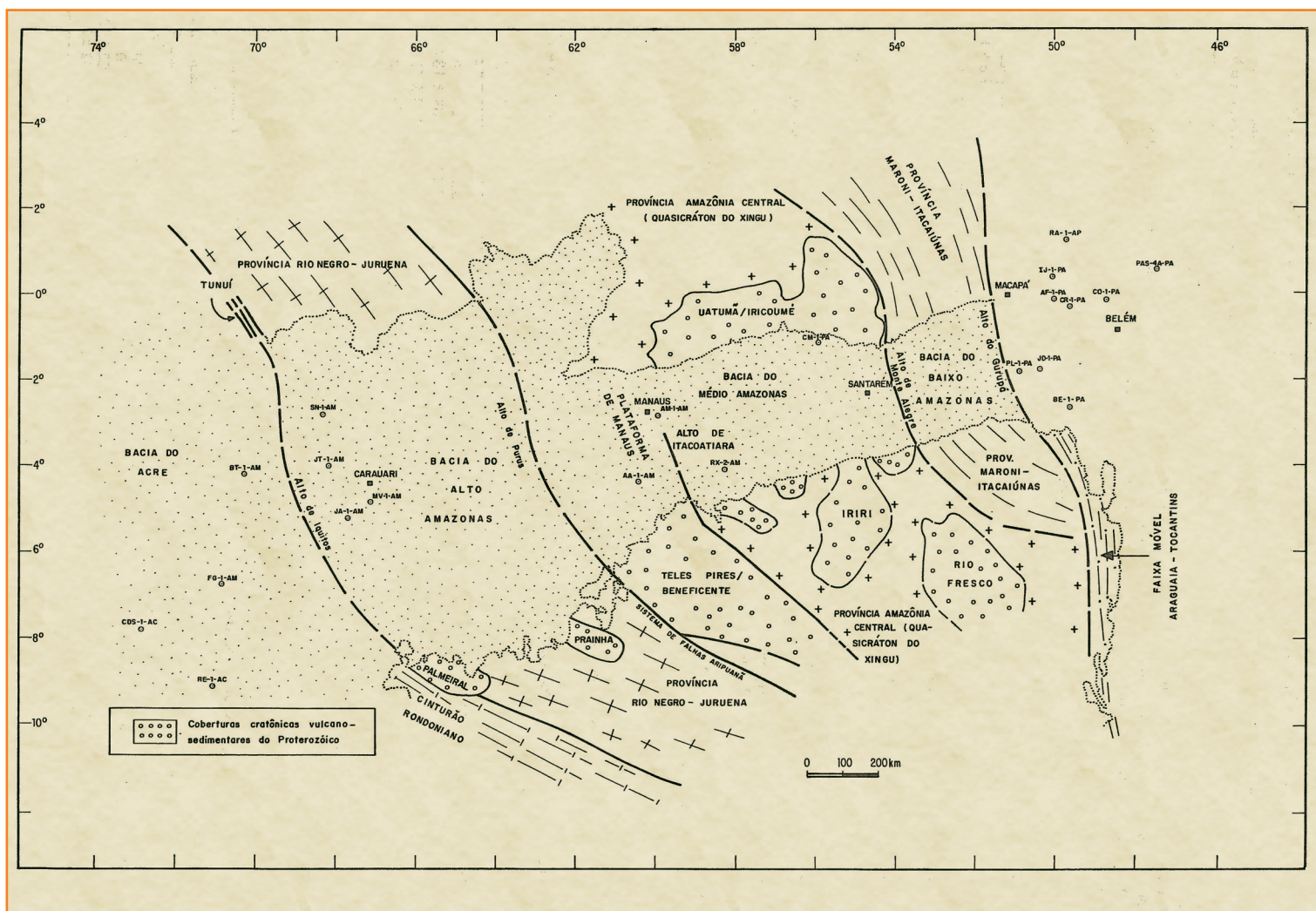
Figura 9 Mapa geológico-geotectônico esquemático do embasamento da Bacia do Amazonas.
