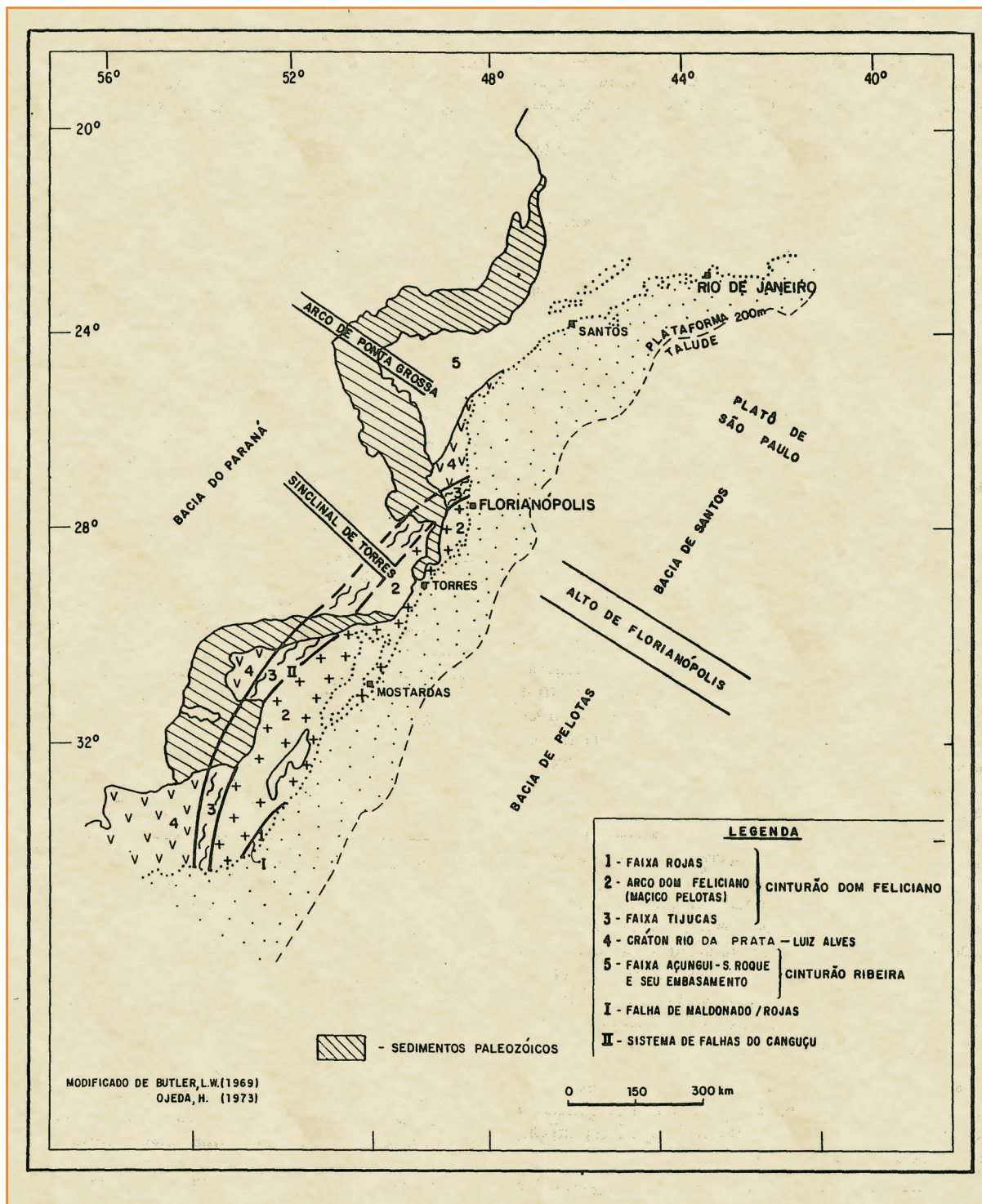
Figura 20 Mapa geológico-geotectônico esquemático do embasamento do Sul/Sudeste do Brasil.
